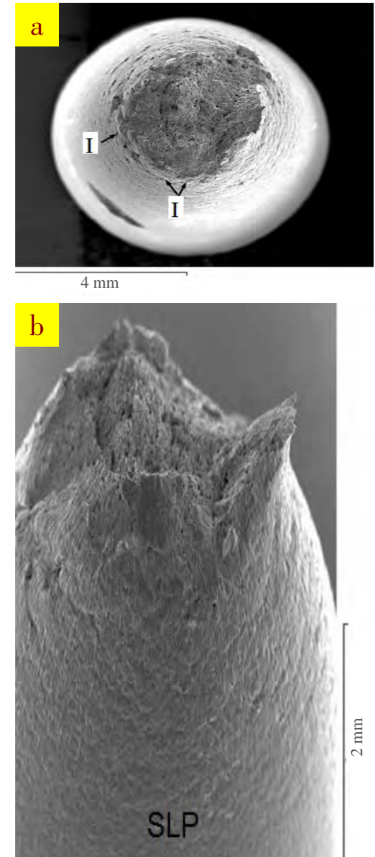
Figura 9. Fotomicrografías obtenidas por MEB (a) Vista general de la superficie de fractura a 15x y (b) Vista general de la superficie de fractura inclinada ~45°, a 25x.
