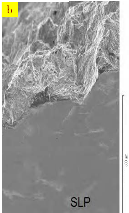
Figura 10. Fotomicrografías obtenidas por MEB de una probeta de Cu con 8 pases por ECAP, ensayado a fatiga a un esfuerzo máximo fluctuante de 210 MPa: (a) Vista general de la superficie de fractura a 15x; (b) Vista de la superficie lateral de la probeta y del inicio de la grieta por fatiga a 100x.
